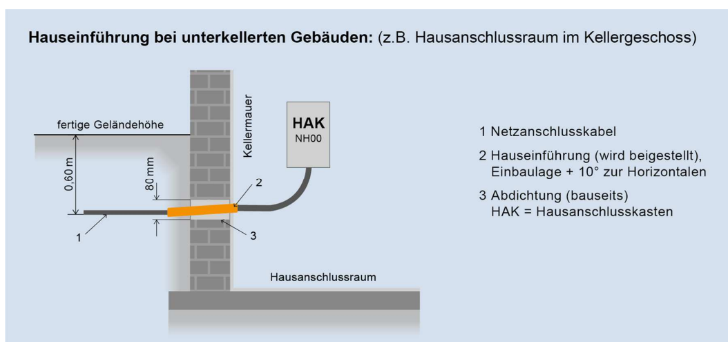
Bild 3: Hauseinführung bei unterkellerten Gebäuden (z. B. Hausanschlussraum im Kellergeschoss)
