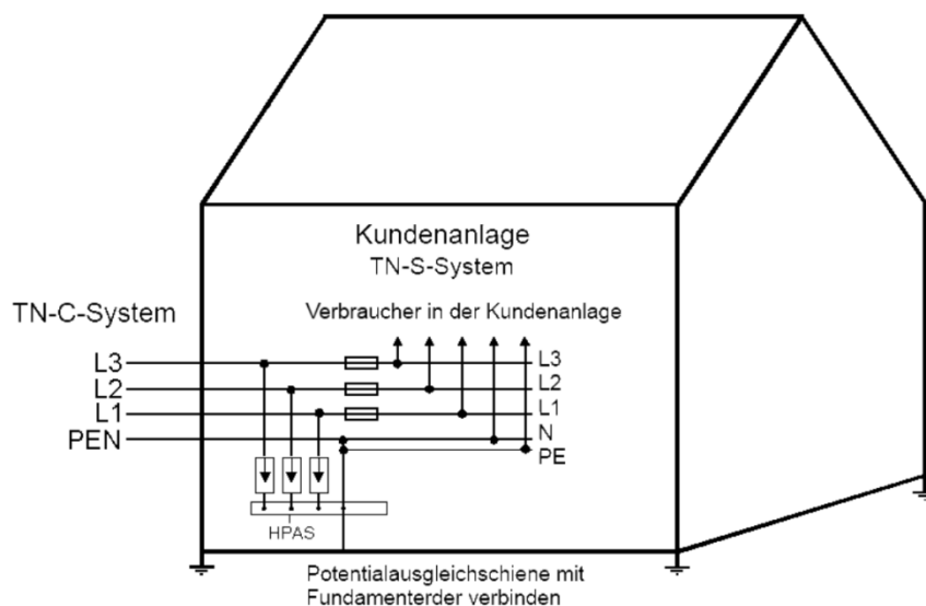
Bild 9: TN-S-System in der Kundenanlage
