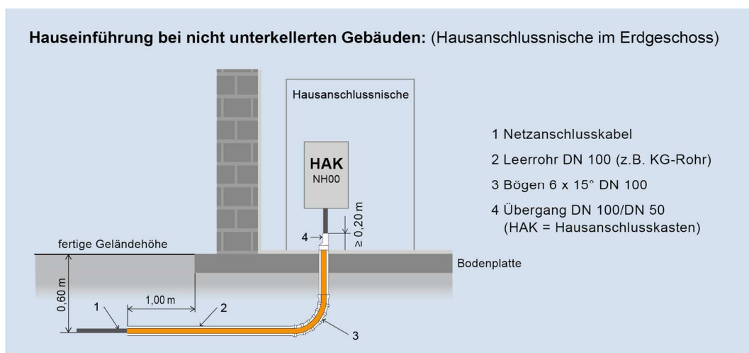
Bild 5: Hauseinführung bei nicht unterkellerten Gebäuden (Hausanschlussnische im Erdgeschoss)
