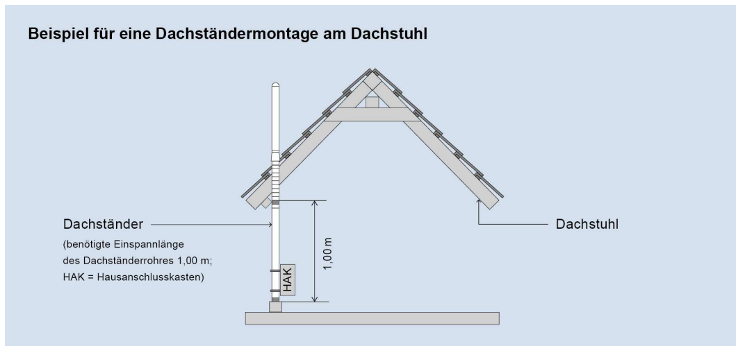
Bild 1: Beispiel für eine Dachständermontage am Dachstuhl
