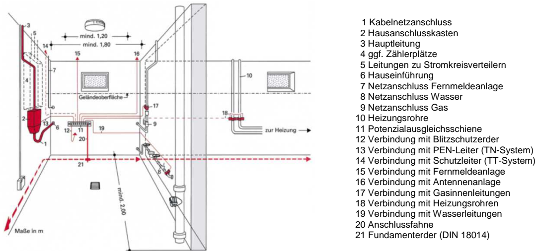
Bild 4: Hausanschlussraum nach DIN 18012 (Quelle: Fachverband Energiemarketing und -Anwendung – HEA)
