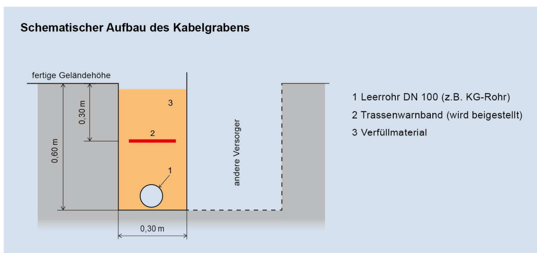
Bild 2: Schematischer Aufbau des Kabelgrabens
