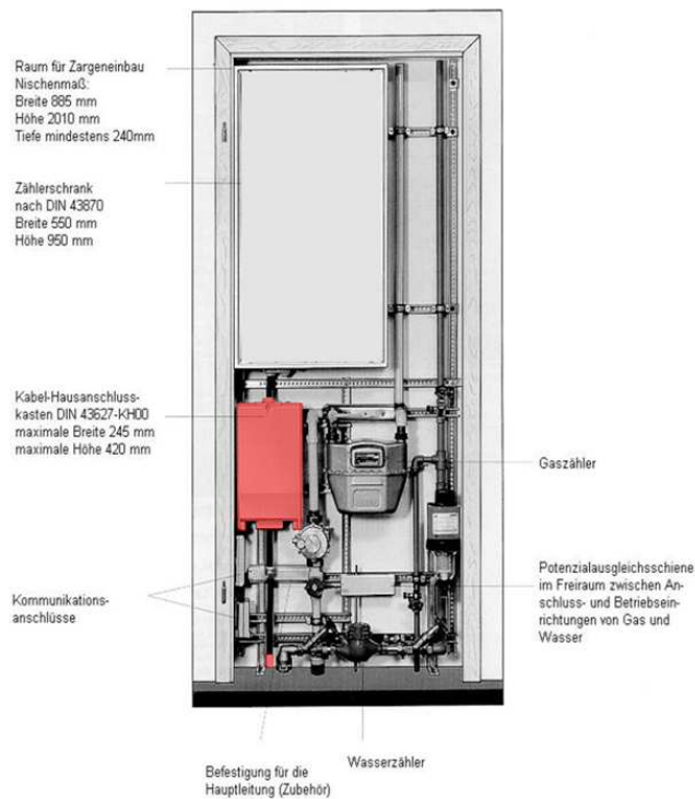
Bild 6: Beispiel für eine Hausanschlussnische (Quelle: Fachverband Energiemarketing und -Anwendung – HEA)
